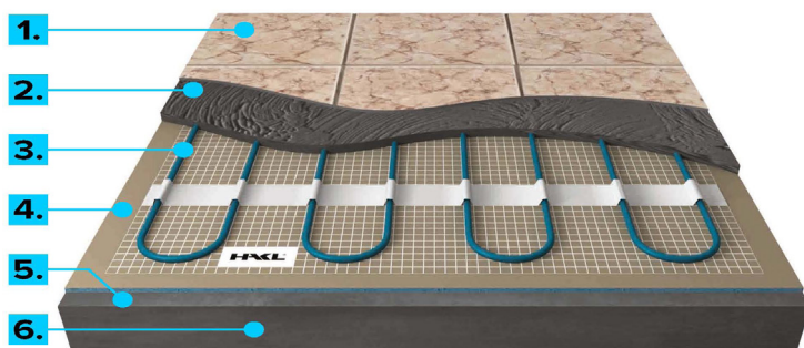
Ilustrační obrázek složení podlahy
