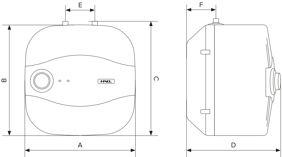
obr. 3: popis rozměrů pro montáž.
